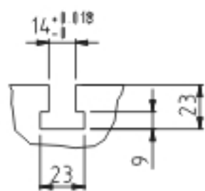
A-View
